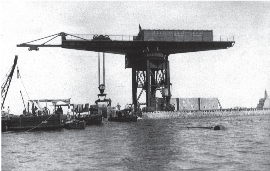
La grúa “Titán” colocando bloques en las obras del Rompeolas de la Isla Verde. Luego quedó varada en mitad del dique que había contribuido a construir a cuya sombra pescaba Rafael Matoso en 1954.
