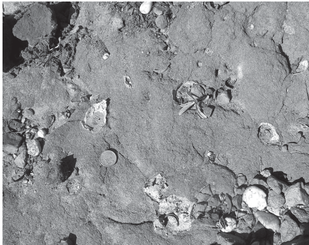
Área de Punta Mala. Terrazas marinas escalonadas.
